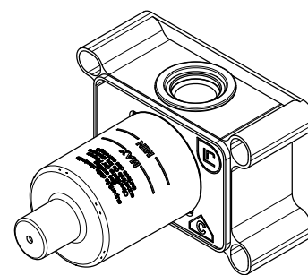
Vista ISO
