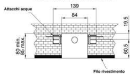
SCHEMA DIMENSIONALE (VISTO DALL'ALTO)
