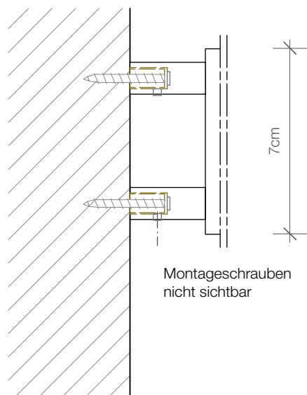
Schnitt Section
